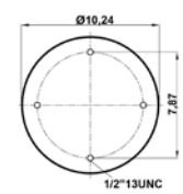
PISTON BOTTOM
