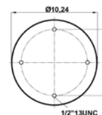
PISTON BOTTOM
