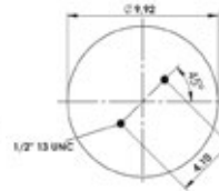
PISTON BOTTOM
