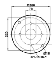
PISTON BOTTOM
