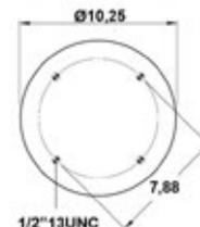
PISTON BOTTOM
