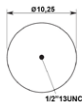
PISTON BOTTOM
