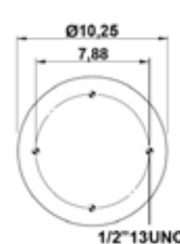
PISTON BOTTOM
