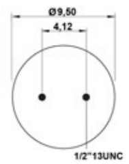
PISTON BOTTOM
