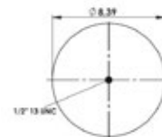
PISTON BOTTOM
