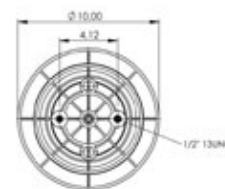
PISTON BOTTOM
