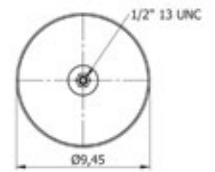
PISTON BOTTOM
