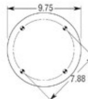
PISTON BOTTOM
