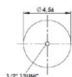
PISTON BOTTOM
