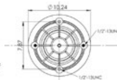
PISTON BOTTOM
