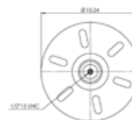
PISTON BOTTOM
